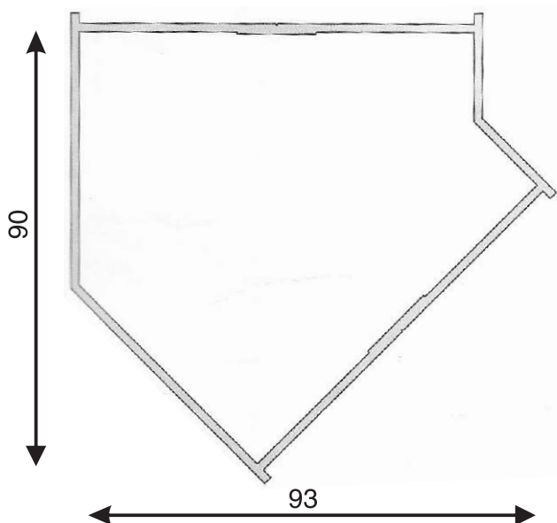
LA 718 Columna acople 45° PESO: 1,312 Kg/m LARGO STD 6030mm
